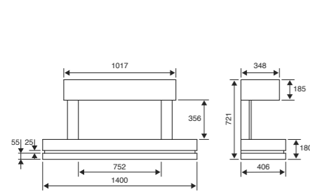
VOLARE 750 ILLUMIA
