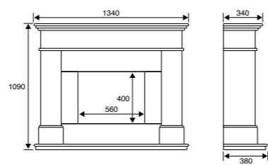
ADOUR ILLUMIA
