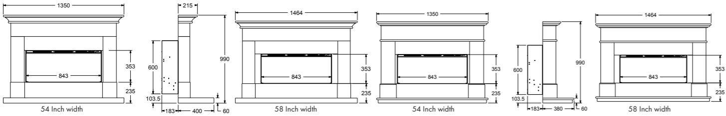
PARADA ELITE ILLUMIA
